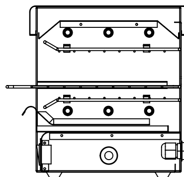
SECCIÓN A-A
