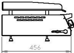
PLC800ECON
